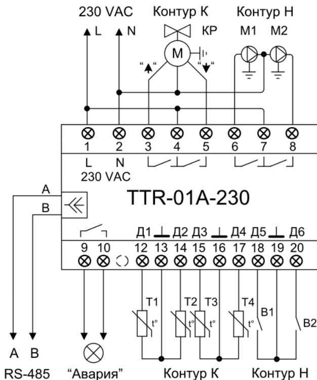
Рисунок В.1 - Схема электрическая подключений ТК-TTR-01A-230
