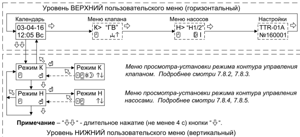
Рисунок 13 - Структура меню настройки режима работы контура
