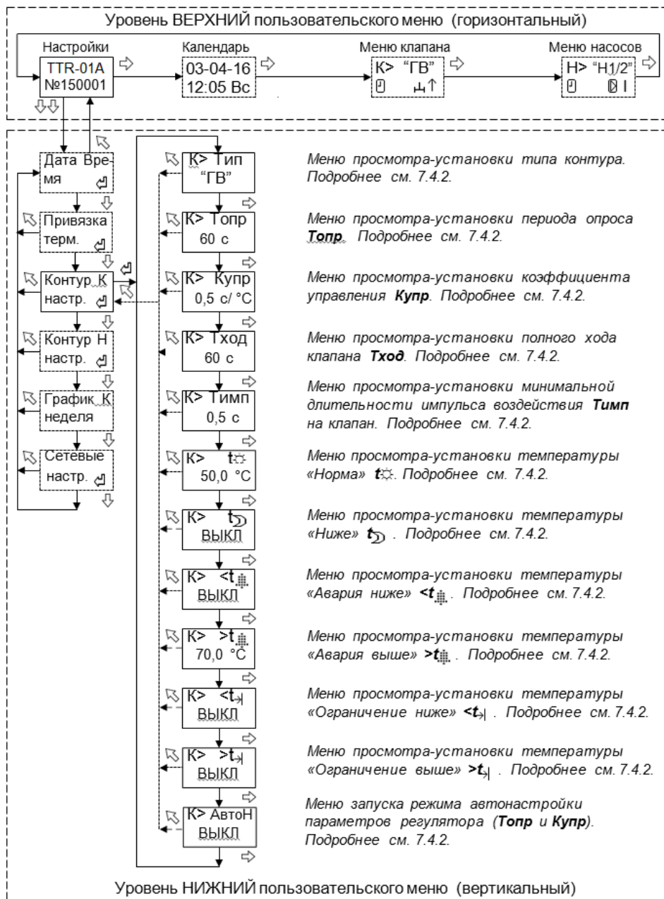
Рисунок 5 - Структура меню настройки параметров контура управления насосами.
